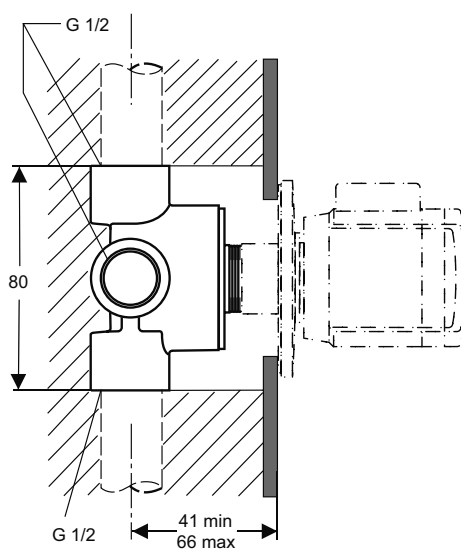
A2391 ..
