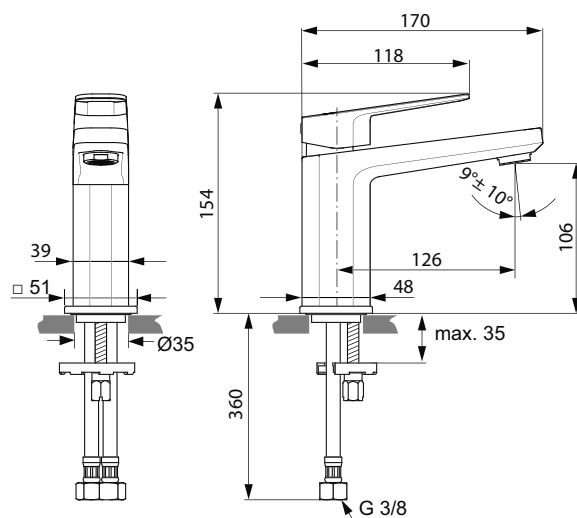
A 6327 ..
