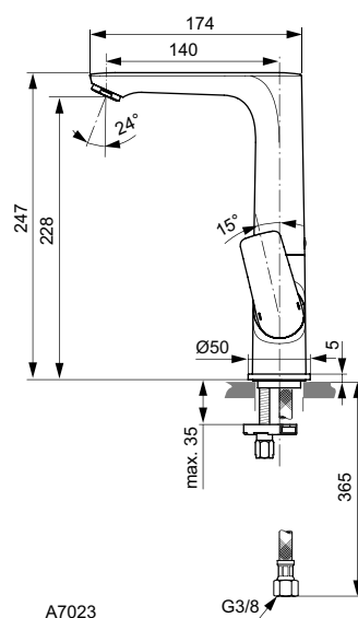
A7023
