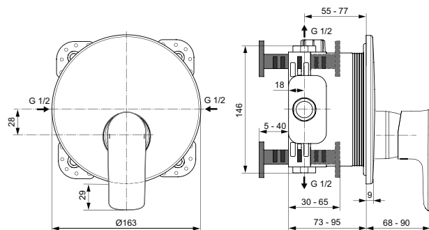
A7034
