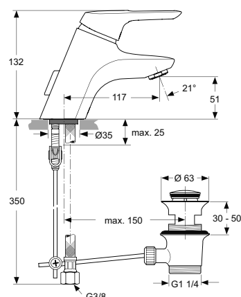
A5651
