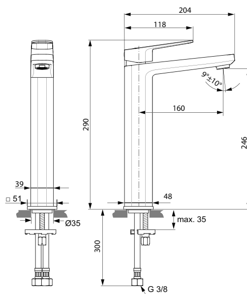
A 6329 ..
