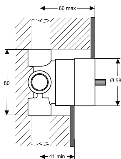
A2393 ..
