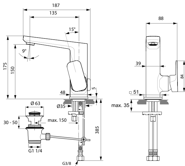
A 6332 ..
