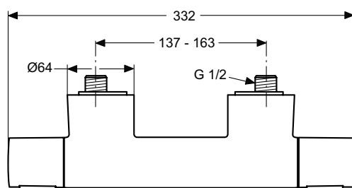
A 4627 ..
