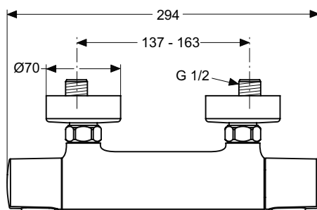
A 4618 ..
