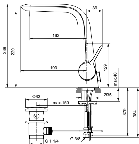
A 6041 ..
