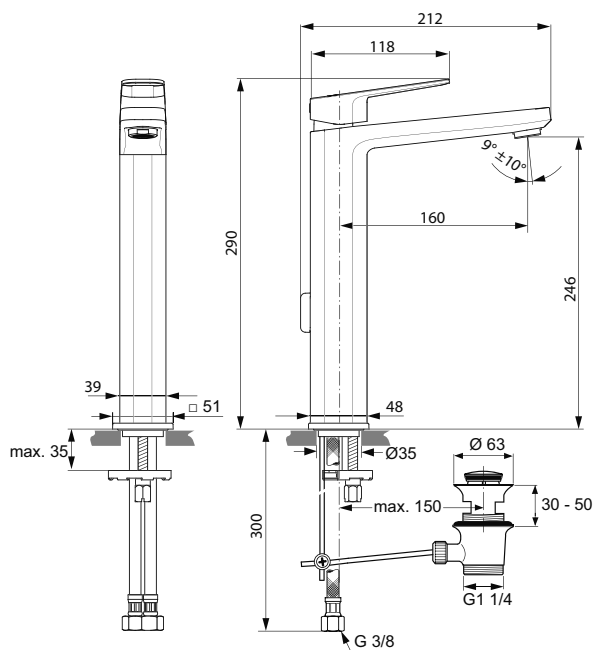
A 6328 ..
