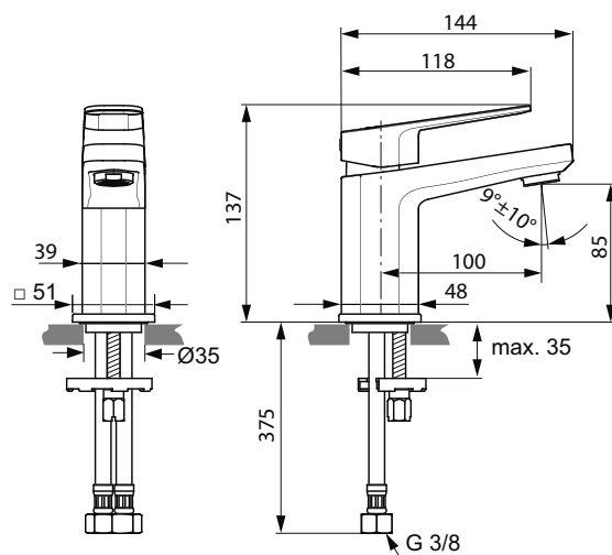
A 6331 ..
