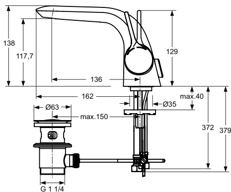
A4260 ..
