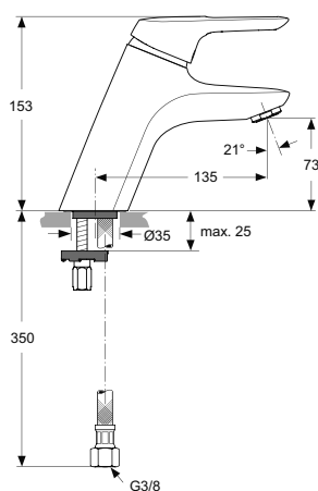
A5647
