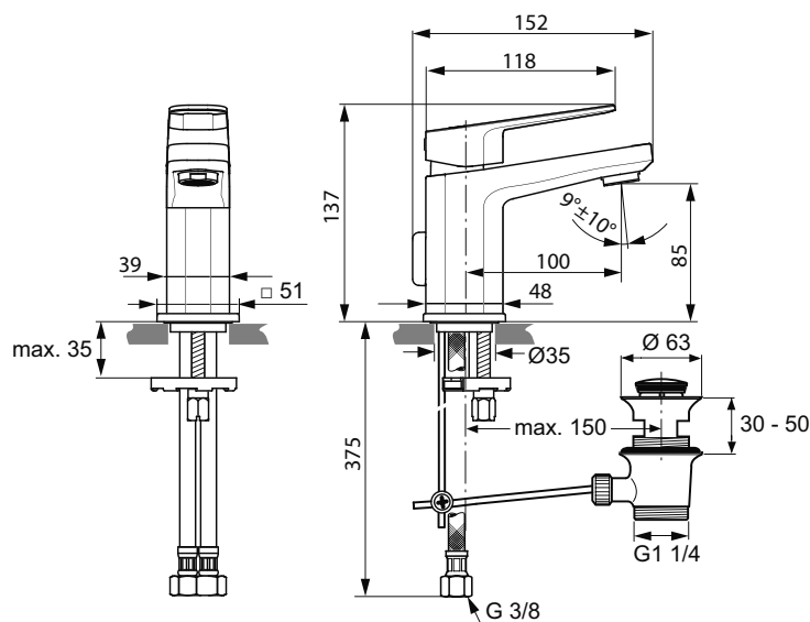
A 6330 ..
